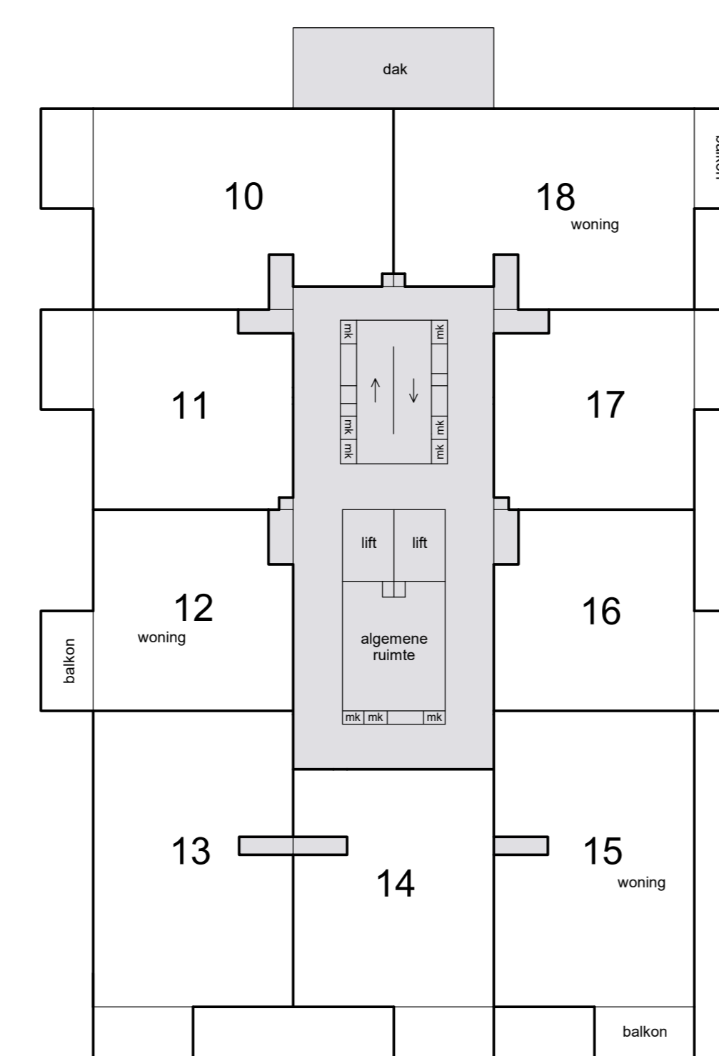
2e etage
