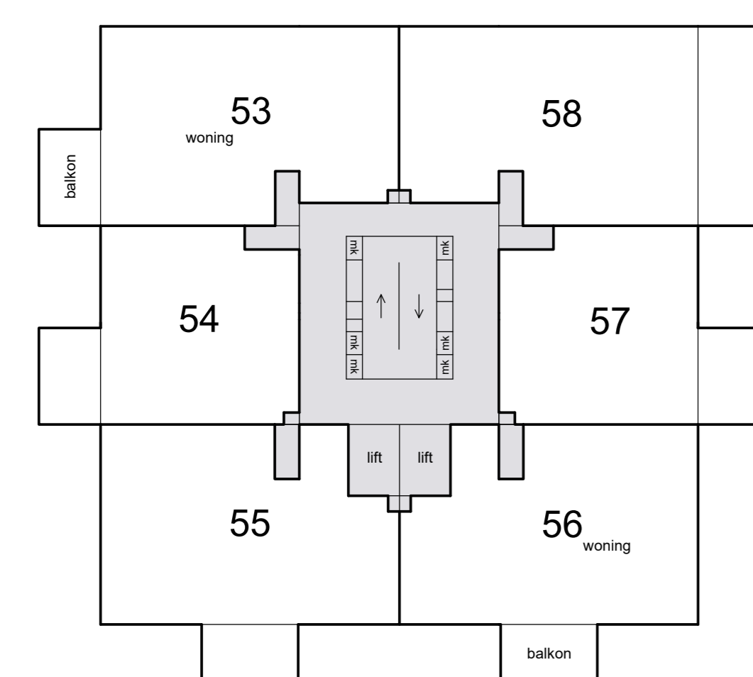
8e etage
